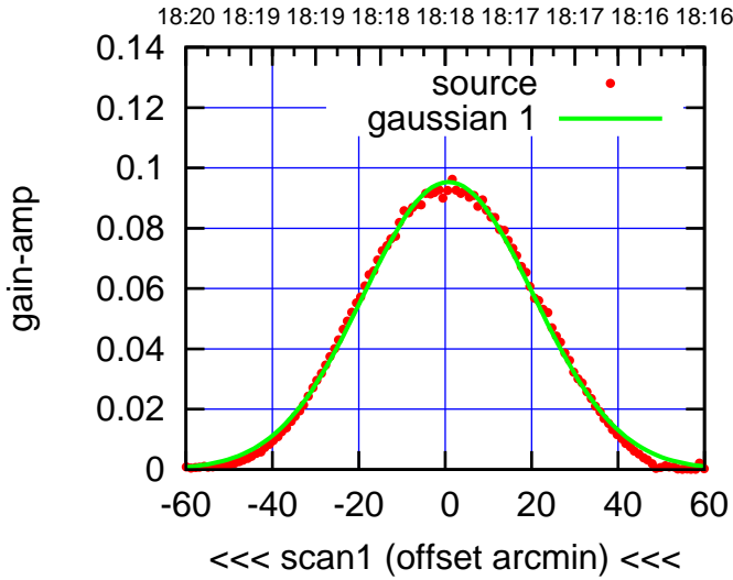
W06-130-AZ OFF= 1.4'
