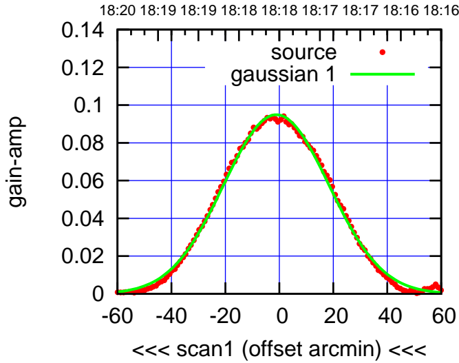
C14-130-AZ OFF= -0.1'
