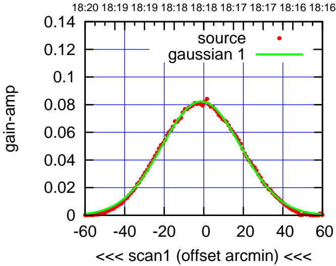
S04-130-AZ OFF= -0.8'
