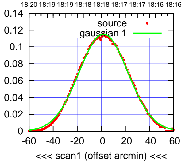
E04-175-AZ OFF= 2.4'
