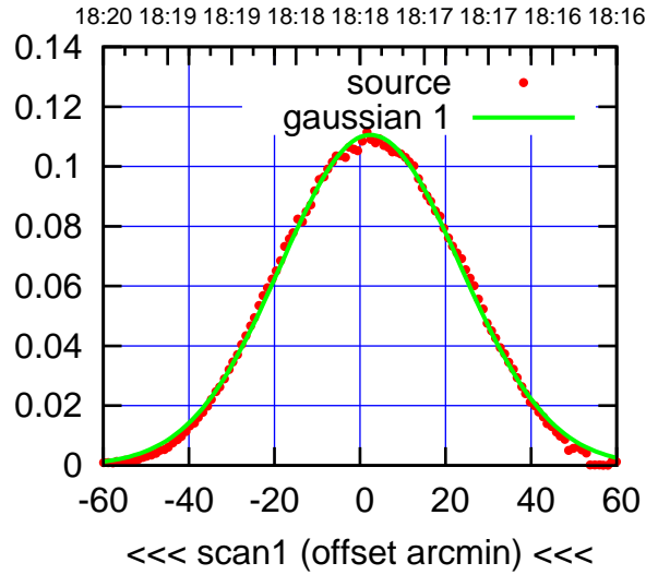
E02-175-AZ OFF= 3.4'
