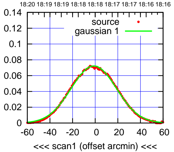
E06-175-AZ OFF= 0.6'
