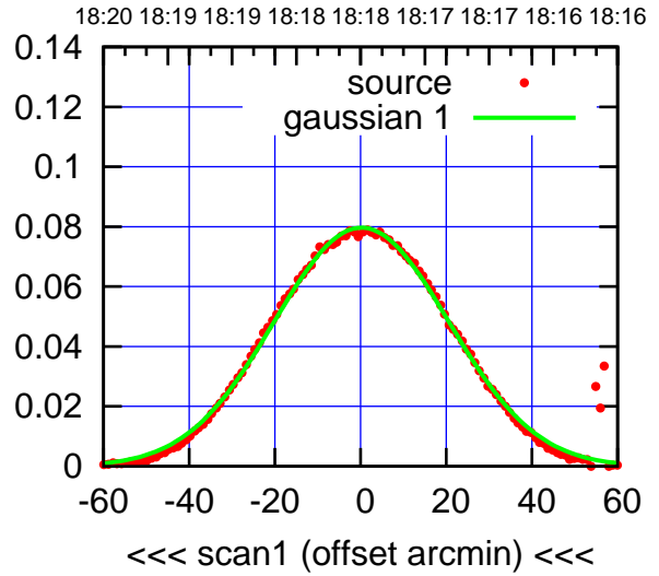
C09-175-AZ OFF= 1.5'
