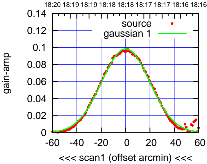
C06-130-AZ OFF= 0.8'
