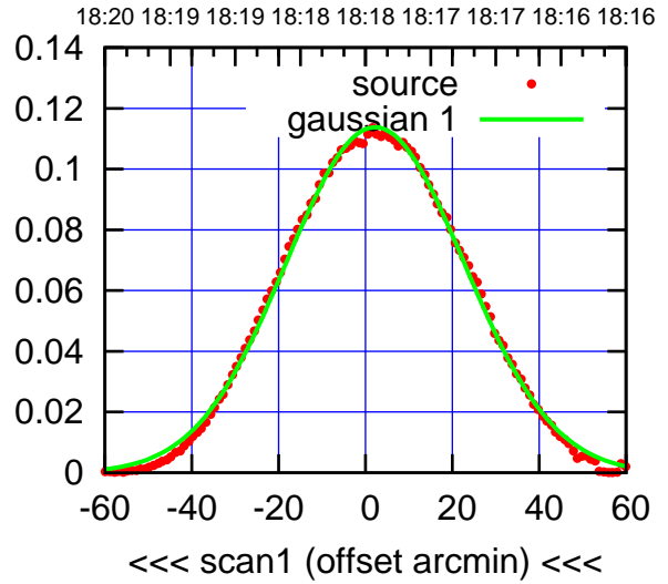
S01-175-AZ OFF= 3.4'
