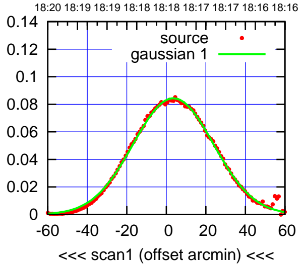
C08-175-AZ OFF= 3.8'
