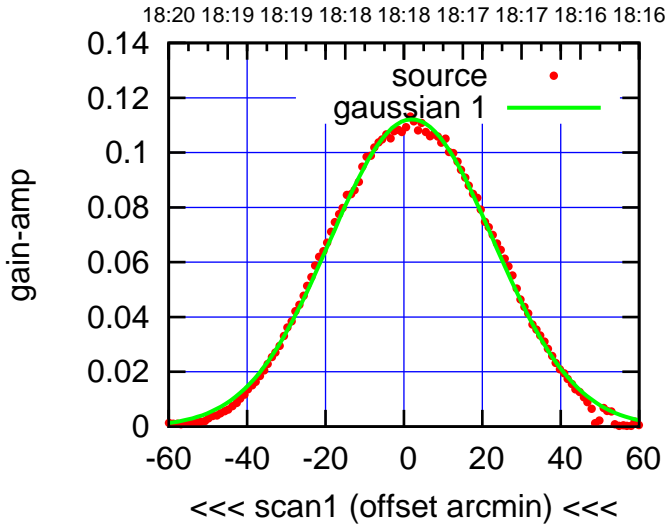
E02-130-AZ OFF= 2.9'
