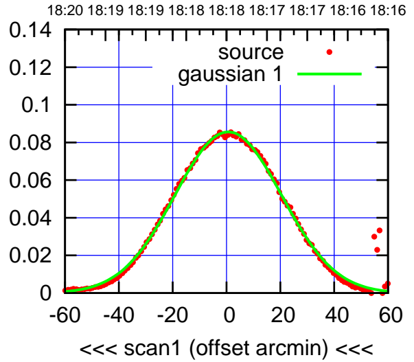
C05-175-AZ OFF= 1.4'
