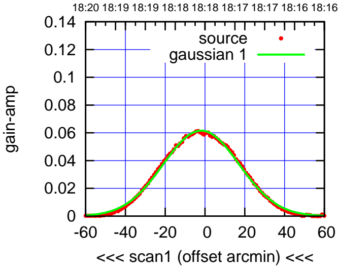
E06-130-AZ OFF= -0.1'
