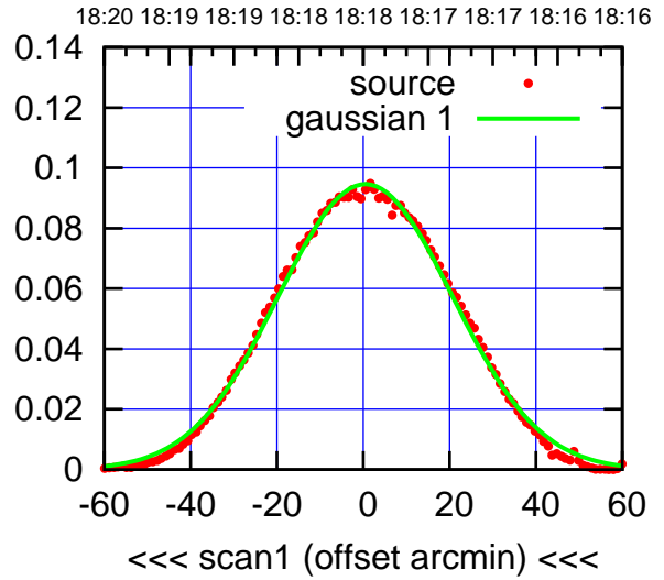
W03-175-AZ OFF= 1.2'
