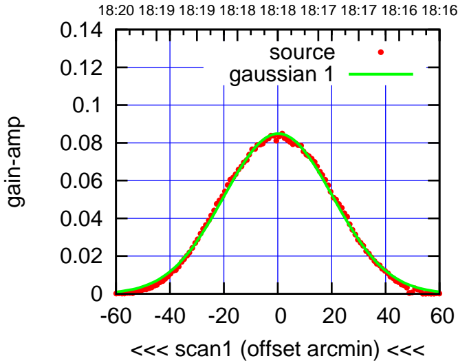
S06-130-AZ OFF= 1.0'
