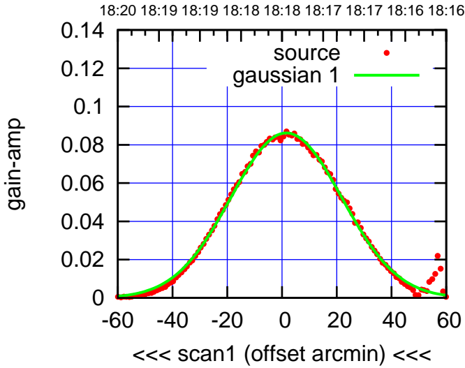
C01-130-AZ OFF= 2.1'
