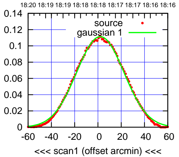
W04-175-AZ OFF= 3.2'
