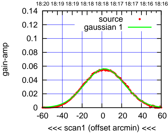
E03-130-AZ OFF= 2.9'
