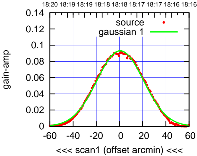
W03-130-AZ OFF= 1.2'
