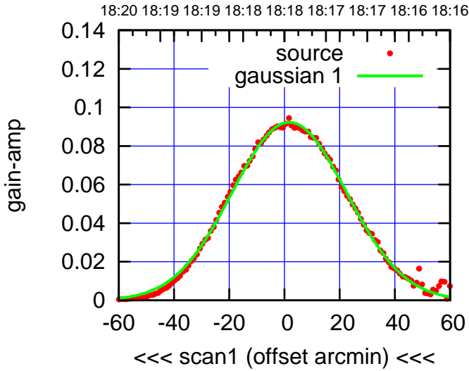
C04-130-AZ OFF= 1.9'
