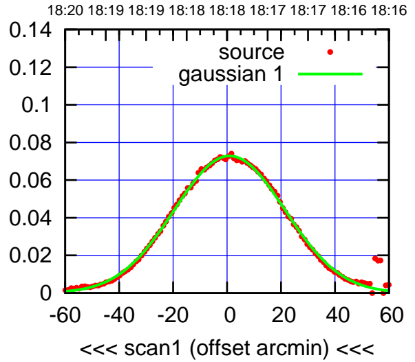
C03-175-AZ OFF= 2.0'
