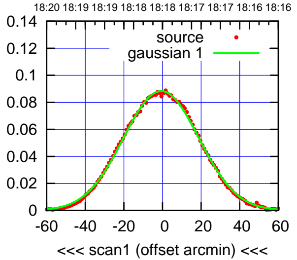
W01-175-AZ OFF= 1.2'
