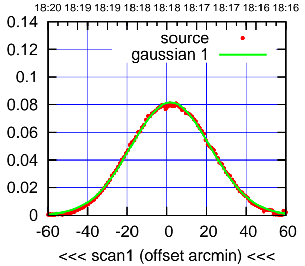
C01-175-AZ OFF= 2.4'
