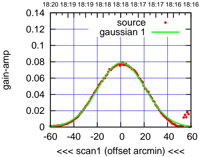
C09-130-AZ OFF= 1.9'
