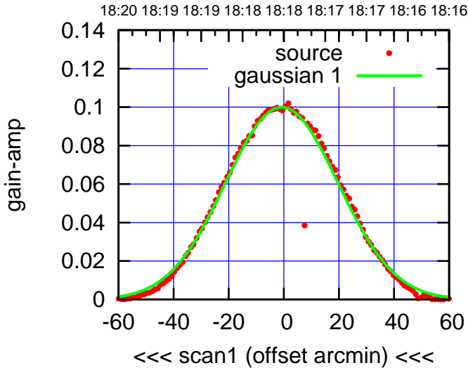
S02-130-AZ OFF= -0.1'
