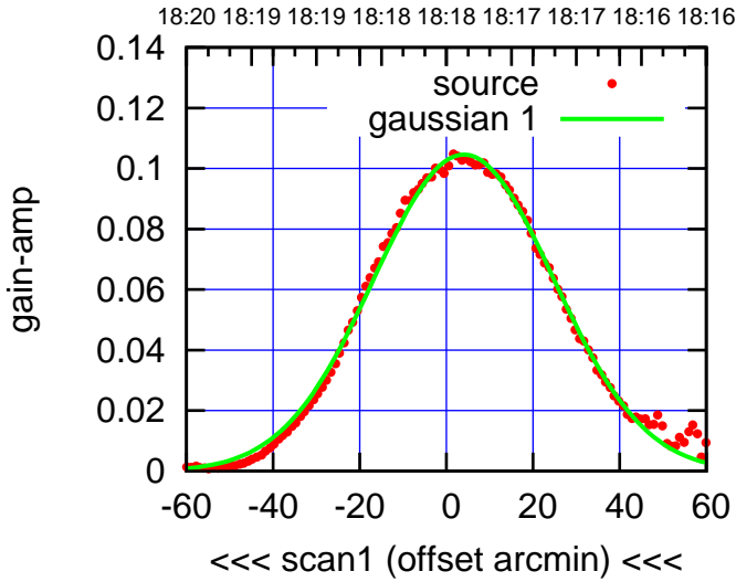
C12-130-AZ OFF= 4.2'
