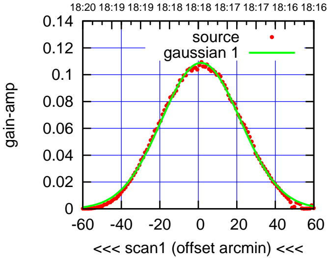
S01-130-AZ OFF= 2.1'
