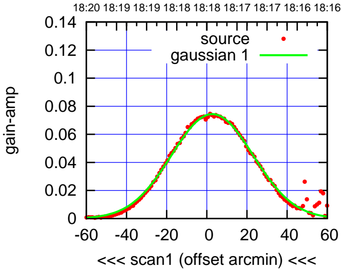
C08-130-AZ OFF= 2.8'
