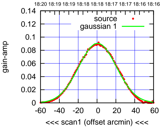
W05-130-AZ OFF= 0.2'
