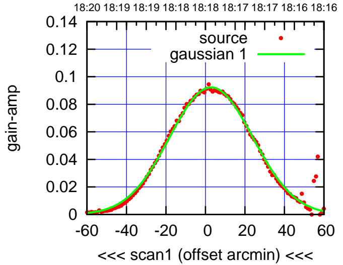
C04-175-AZ OFF= 3.2'
