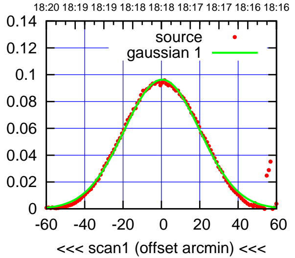
C06-175-AZ OFF= 1.1'
