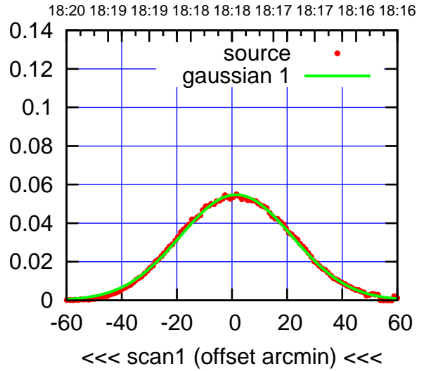
E03-175-AZ OFF= 2.0'
