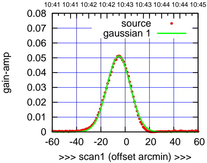
W04-130-EL OFF= -5.1' ( 22.2')
