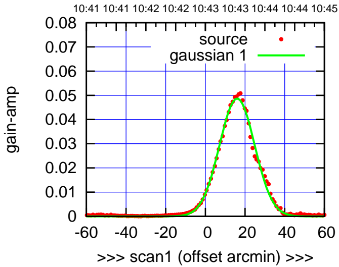
C08-130-EL OFF= 16.2' ( 20.8')
