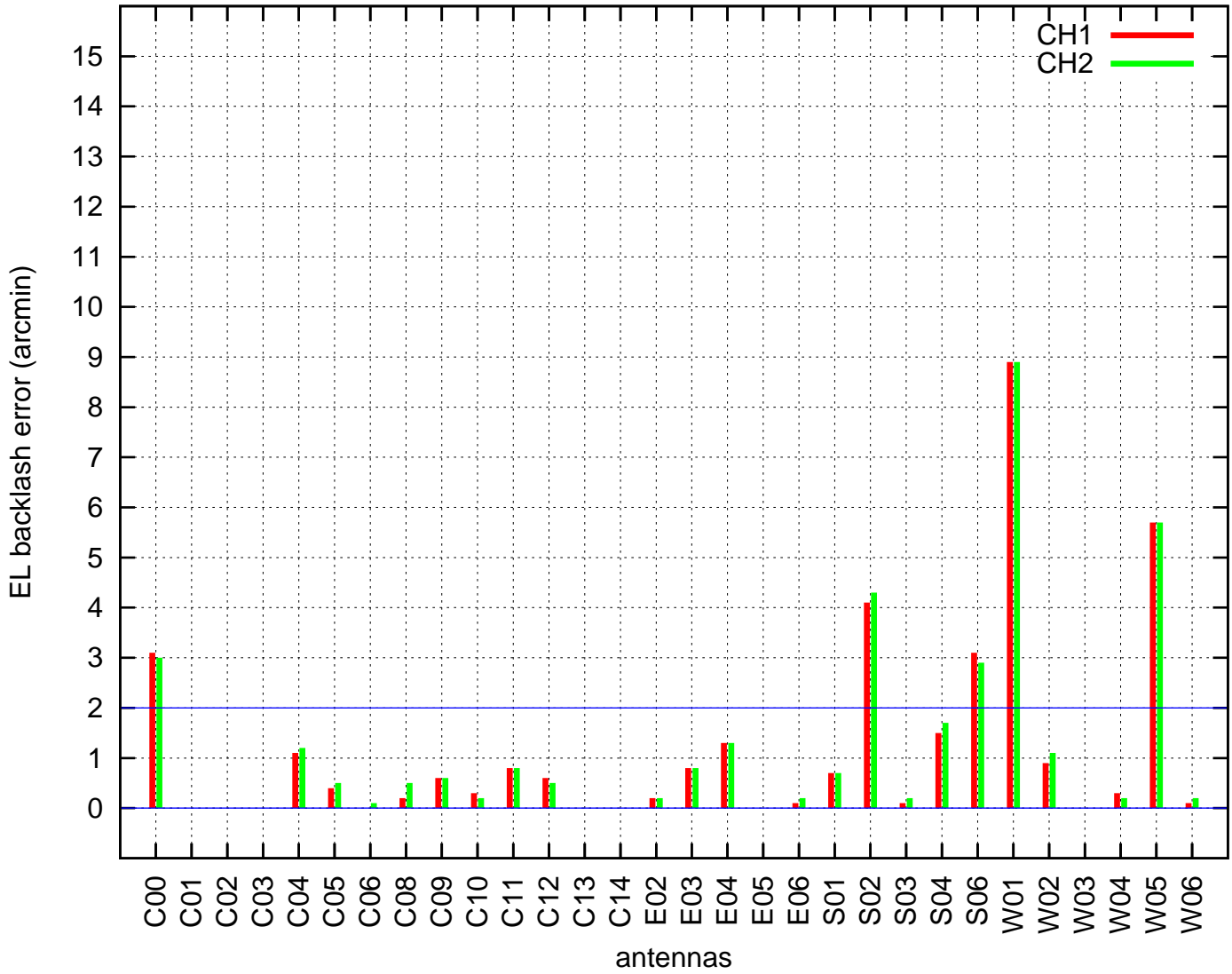
EL backlash test (08Jun2017 10:43:00)
