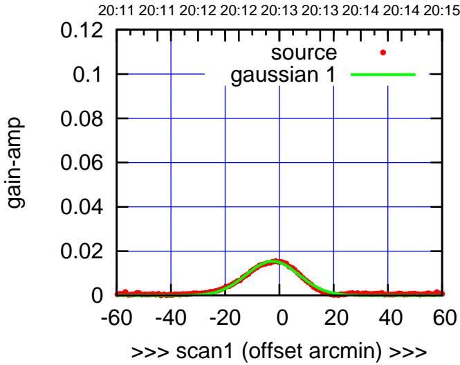
C01-130-EL OFF= 0.6' ( 22.2')
