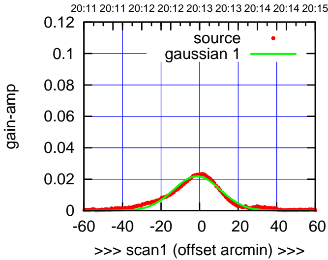
C03-130-EL OFF= -2.0' ( 28.2')
