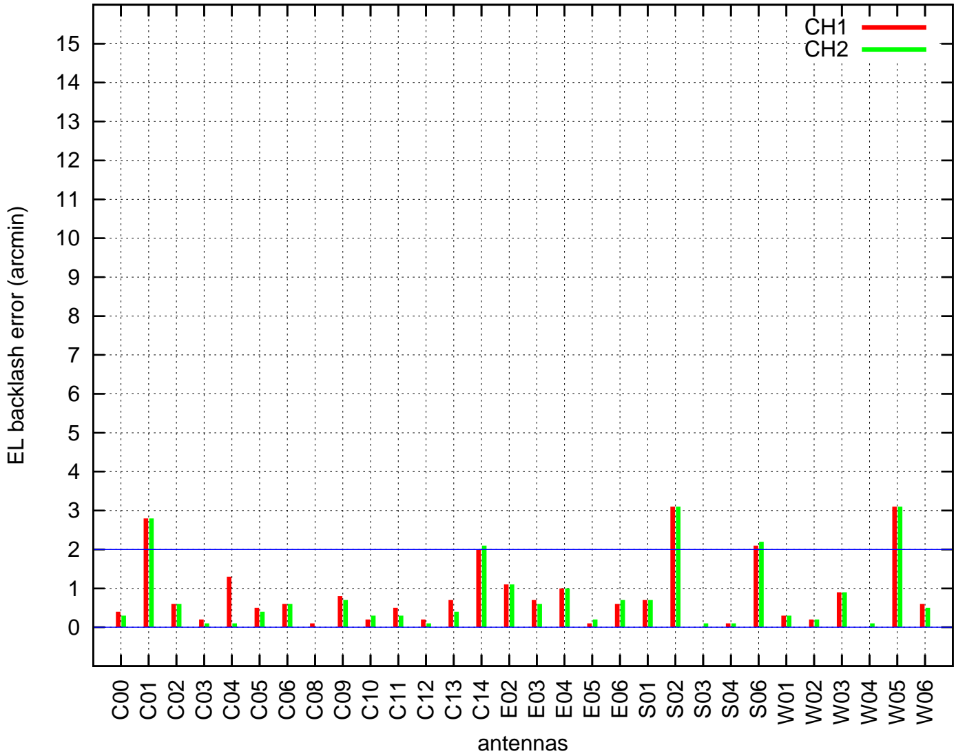
EL backlash test (17Jan2019 22:33:00)
