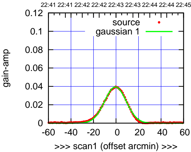
W04-130-EL OFF= -0.7' ( 22.6')
