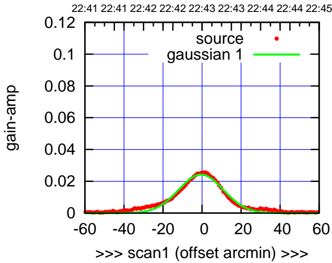
C03-130-EL OFF= -1.0' ( 26.5')
