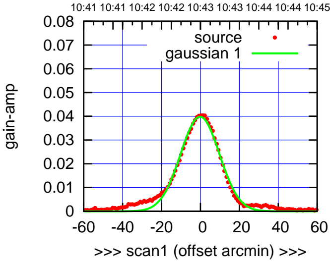
C05-130-EL OFF= -0.7' ( 23.4')
