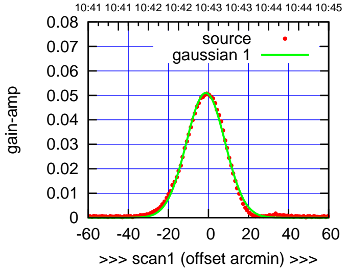
W04-175-EL OFF= -1.0' ( 22.8')
