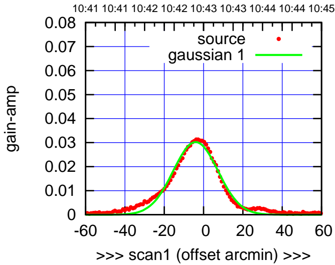
C03-130-EL OFF= -3.9' ( 26.8')
