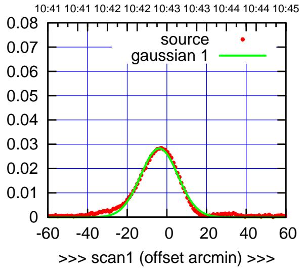
C03-175-EL OFF= -3.7' ( 22.1')
