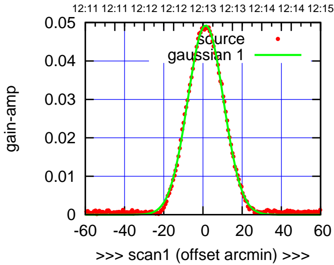
E06-130-AZ OFF= 0.5' ( 21.4')
