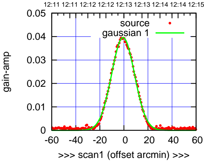
C06-130-AZ OFF= -1.6' ( 22.3')
