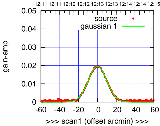
C13-130-AZ OFF= -1.0' ( 23.0')
