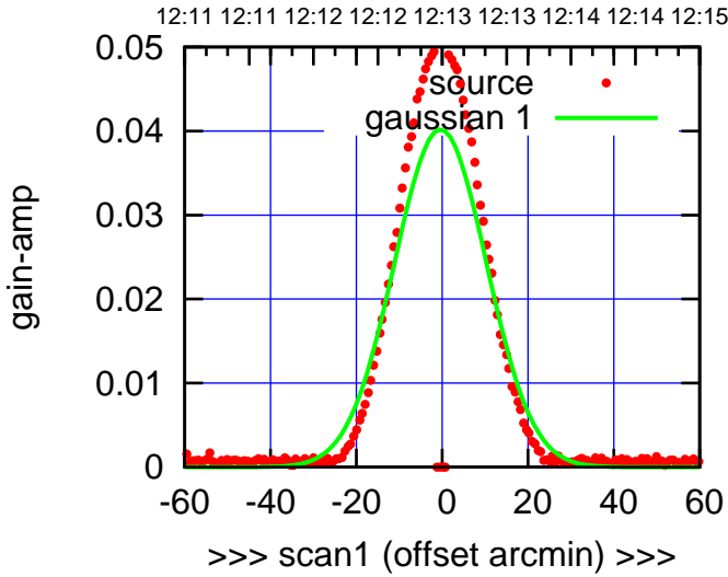
E04-130-AZ OFF= -1.2' ( 26.0')
