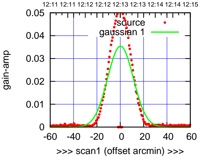
W03-130-AZ OFF= -0.5' ( 26.0')
