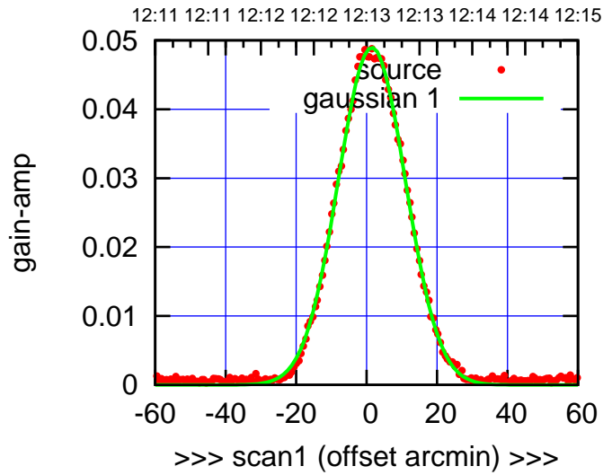
E06-175-AZ OFF= 0.6' ( 23.3')
