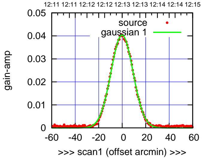
E04-175-AZ OFF= -1.1' ( 22.0')
