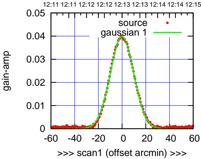
W04-130-AZ OFF= -0.9' ( 23.2')
