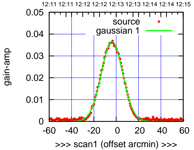
C09-175-AZ OFF= -4.6' ( 22.4')
