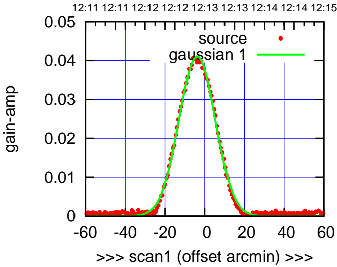
C09-130-AZ OFF= -4.7' ( 21.3')
