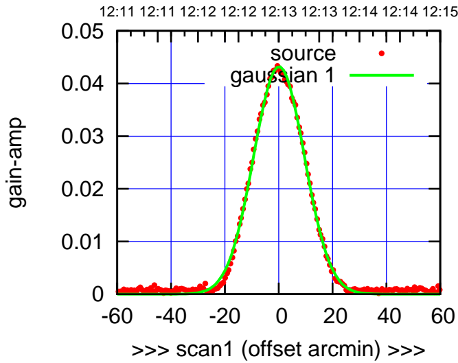
C10-130-AZ OFF= -0.7' ( 22.1')
