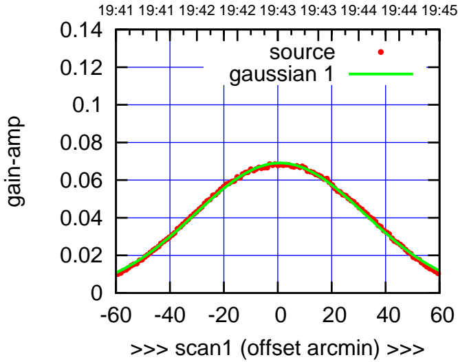
E05-130-AZ OFF= -0.0'
