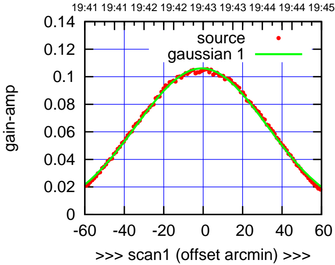
S02-130-AZ OFF= -1.1'
