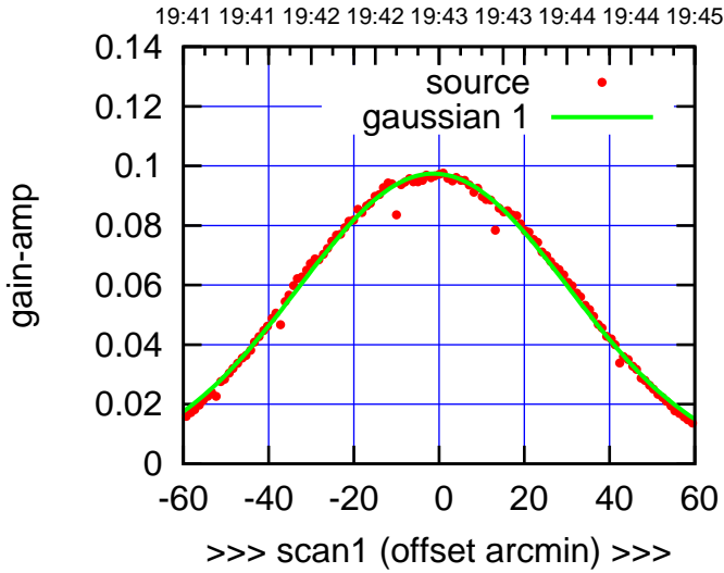
C14-130-AZ OFF= -2.5'
