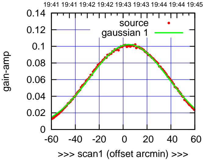
S01-130-AZ OFF= 3.4'
