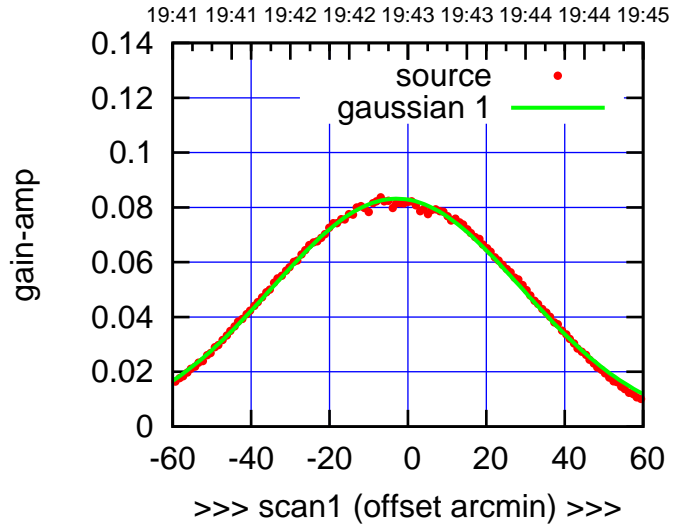
C01-175-AZ OFF= -3.2'
