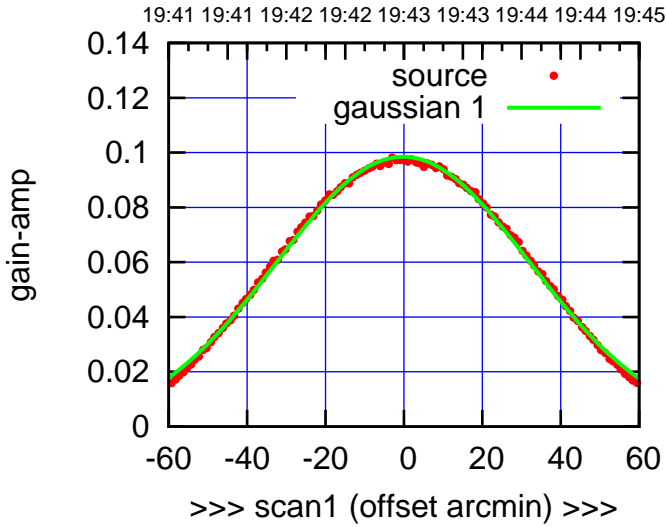
E04-130-AZ OFF= -1.1'
