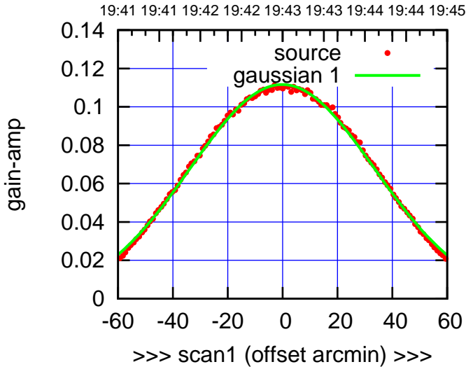
S03-130-AZ OFF= -1.4'
