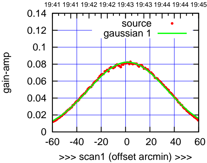
C05-130-AZ OFF= 0.6'
