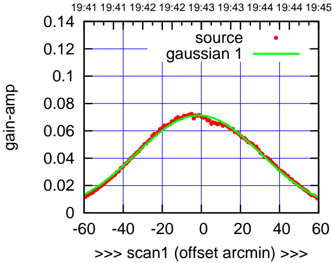
C08-130-AZ OFF= 0.6'
