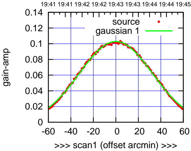
C11-130-AZ OFF= -0.7'
