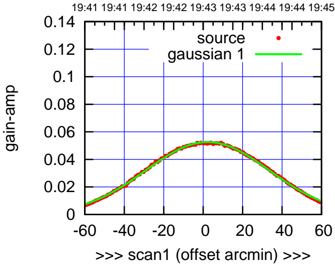
E03-130-AZ OFF= 1.4'
