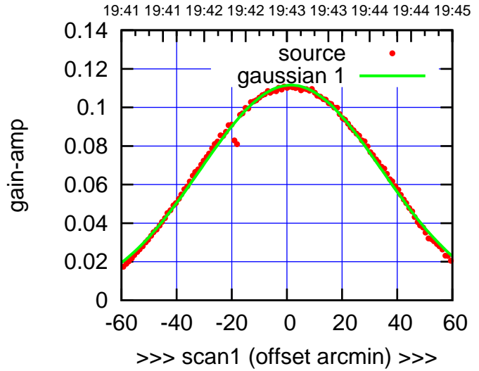
W04-175-AZ OFF= 0.7'
