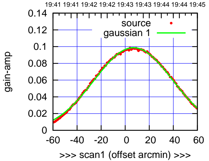
C04-175-AZ OFF= 6.3'
