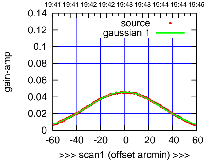
E03-175-AZ OFF= -1.0'
