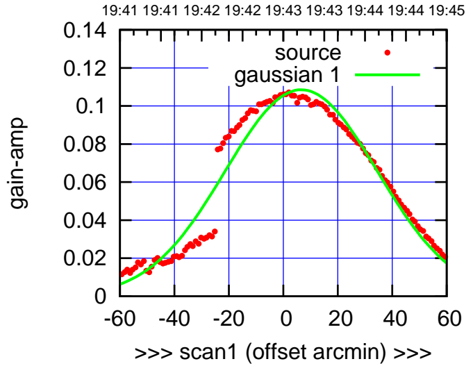
C06-175-AZ OFF= 9.4'
