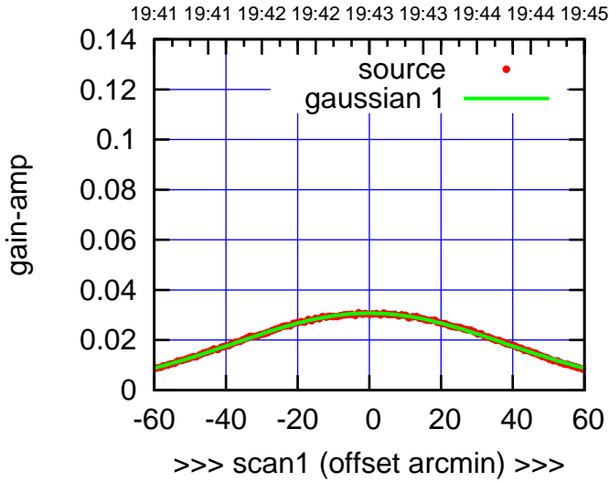
E06-130-AZ OFF= -1.0'
