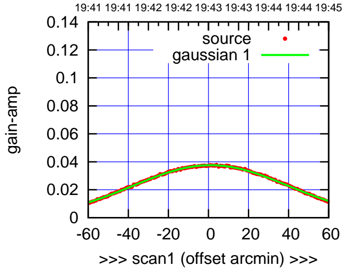
E06-175-AZ OFF= 0.2'
