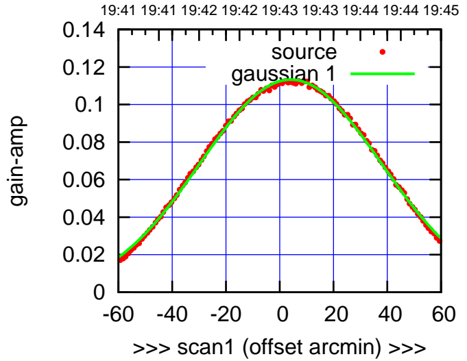
E02-175-AZ OFF= 3.0'
