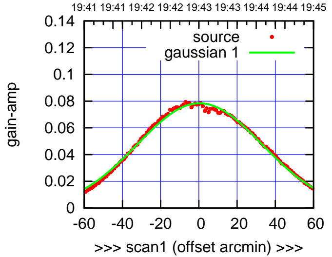
C08-175-AZ OFF= 2.4'
