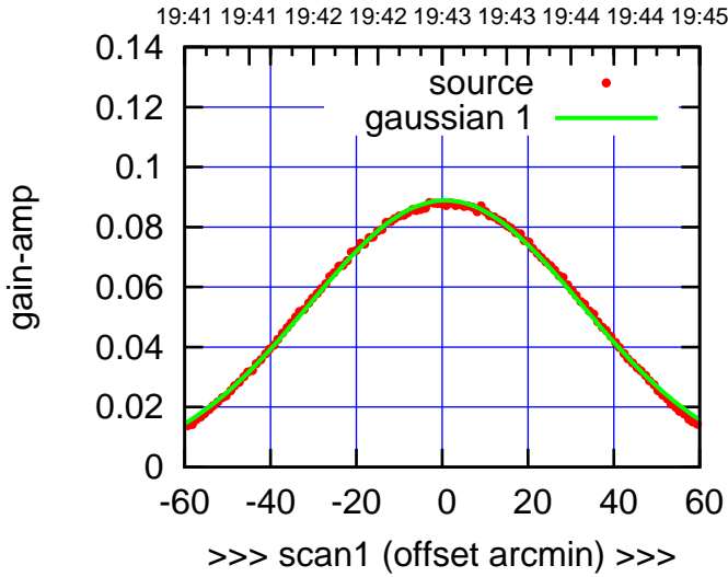
W05-130-AZ OFF= 0.2'
