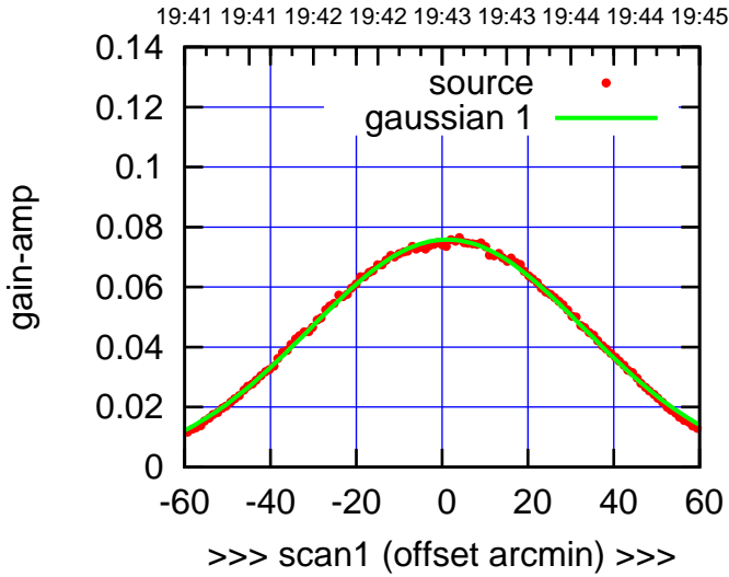
C09-130-AZ OFF= -0.2'
