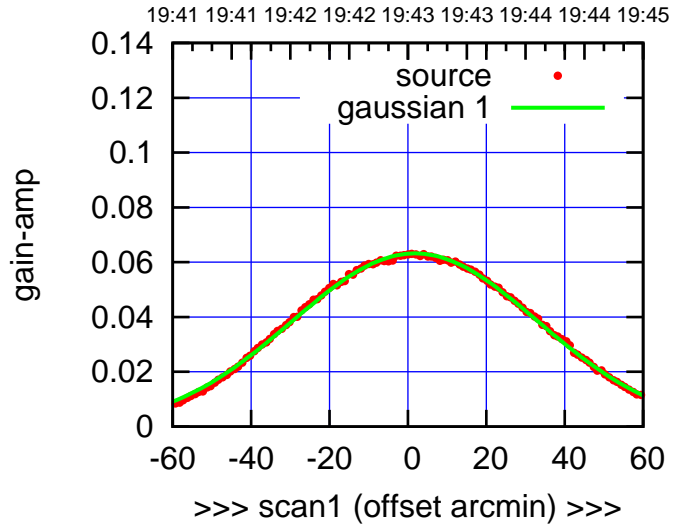
C03-175-AZ OFF= 0.5'
