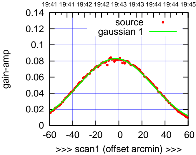
C01-130-AZ OFF= -3.4'
