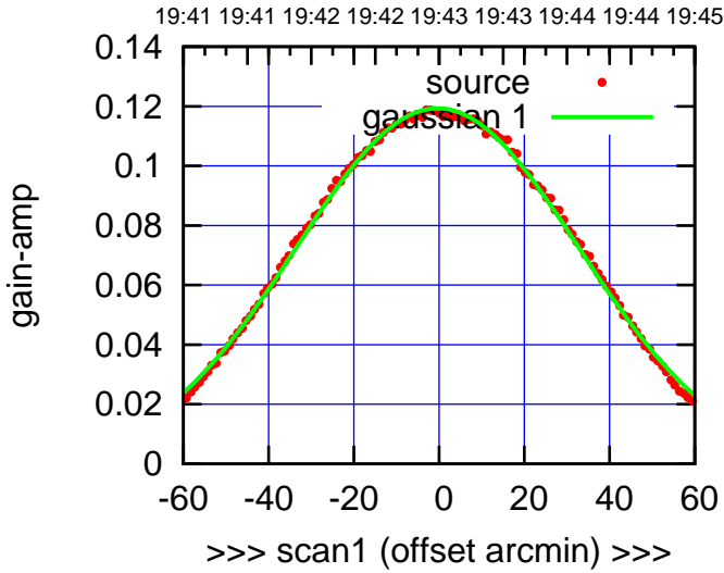
W01-130-AZ OFF= -1.5'
