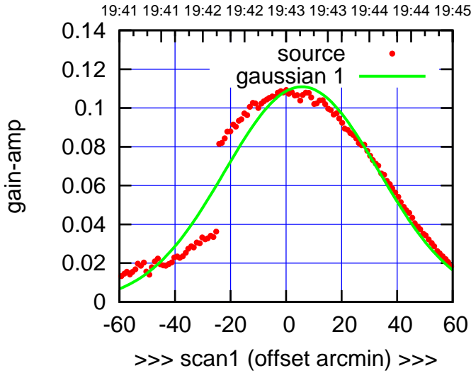
C06-130-AZ OFF= 8.6'
