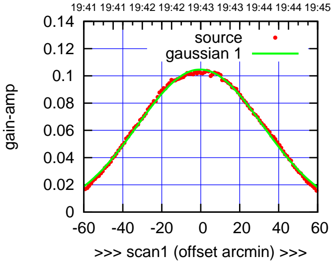
C13-130-AZ OFF= -1.2'
