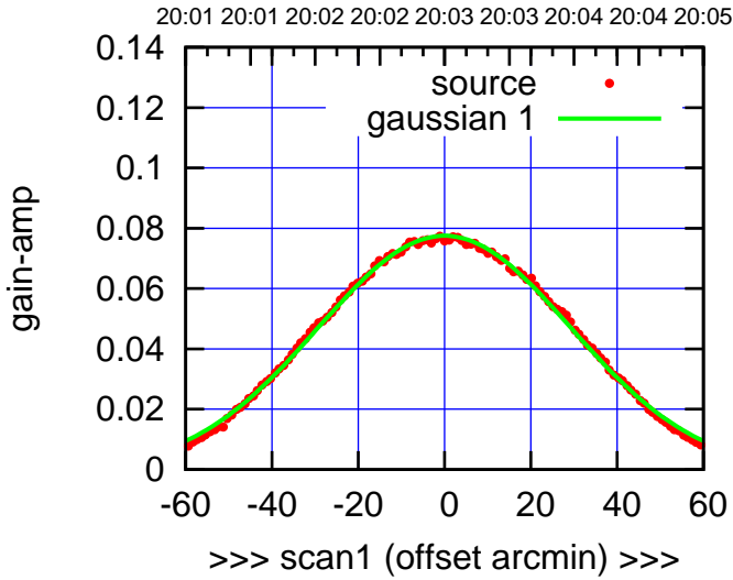
C08-130-AZ OFF= -0.1'
