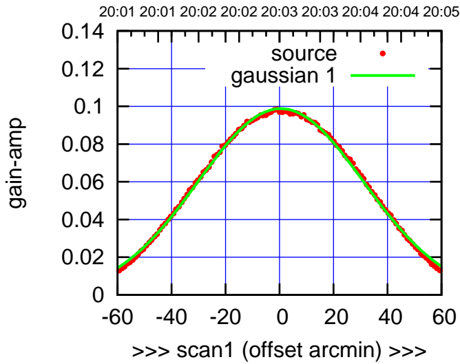
W03-130-AZ OFF= 0.0'
