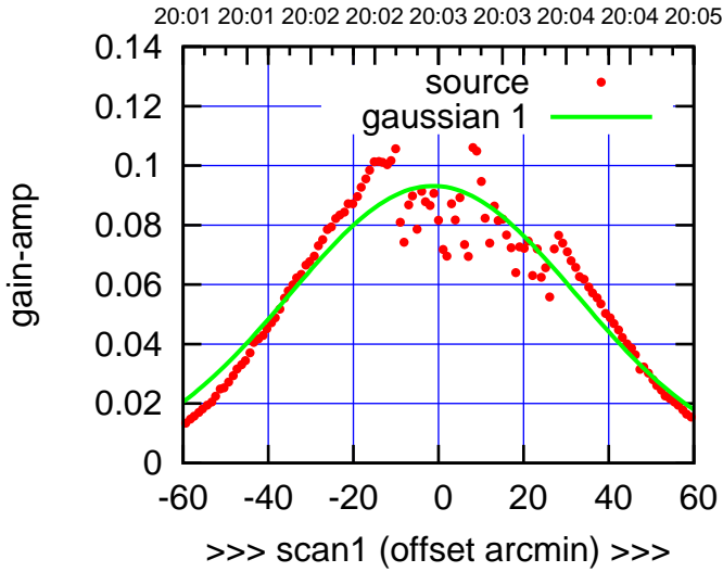
C06-130-AZ OFF= -6.3'
