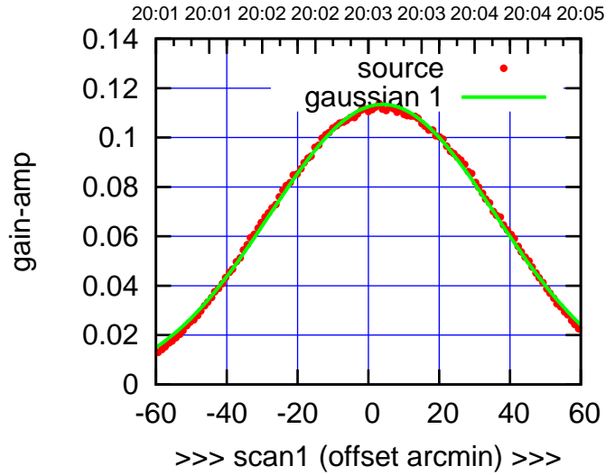
E02-175-AZ OFF= 3.2'
