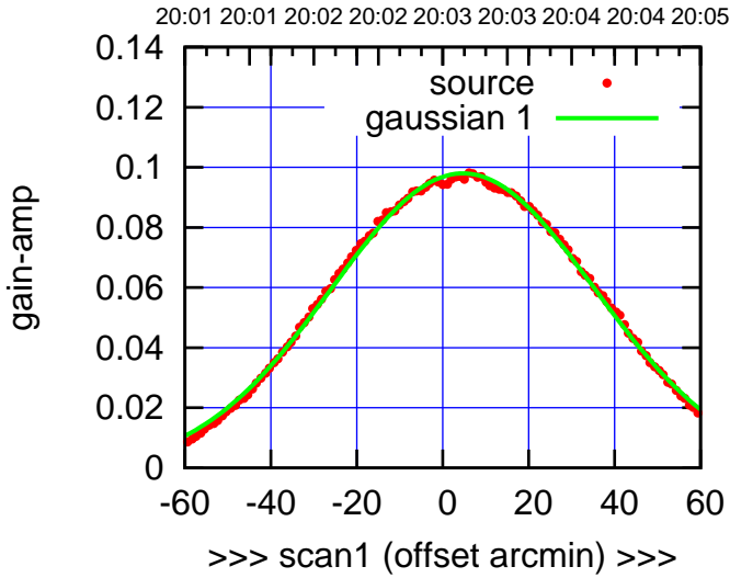
W06-130-AZ OFF= 4.4'
