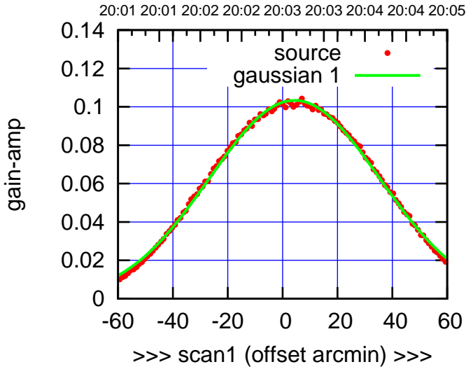
S01-130-AZ OFF= 3.6'
