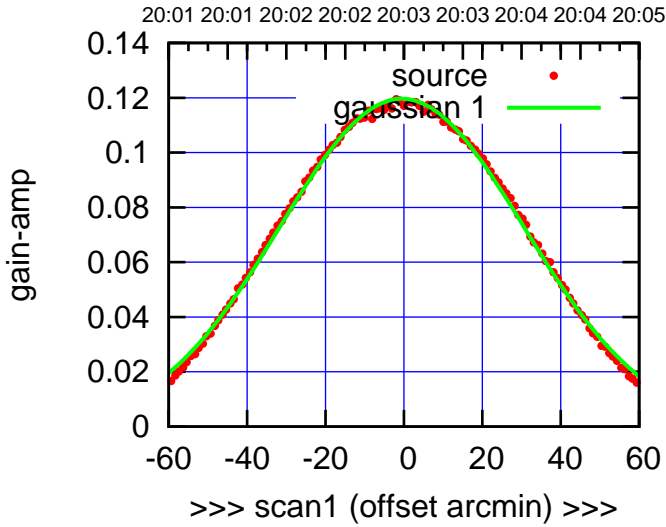
W01-130-AZ OFF= -1.0'
