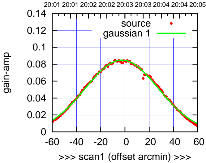
C01-130-AZ OFF= -2.3'
