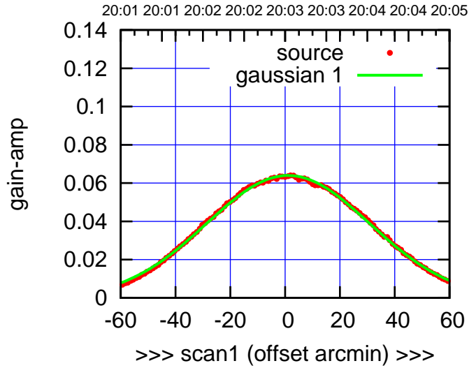
C03-175-AZ OFF= 0.6'
