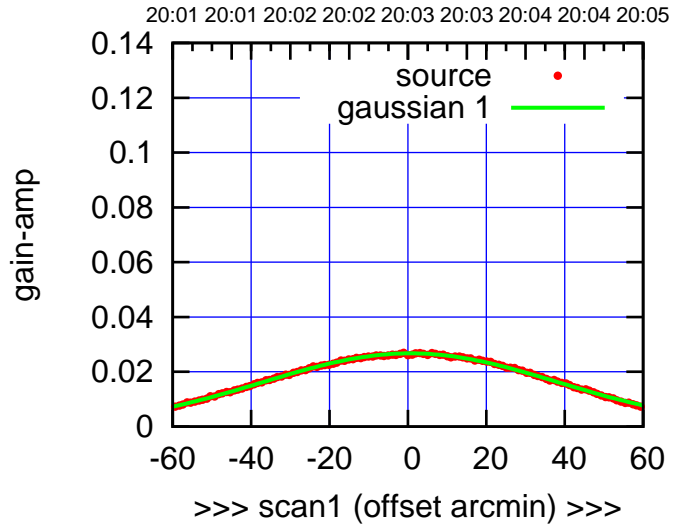
E06-175-AZ OFF= -2.1'
