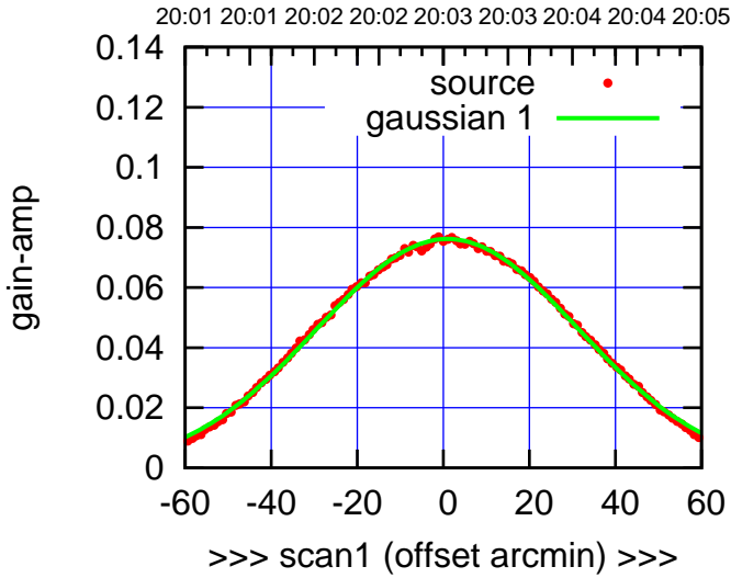
C09-130-AZ OFF= 0.5'
