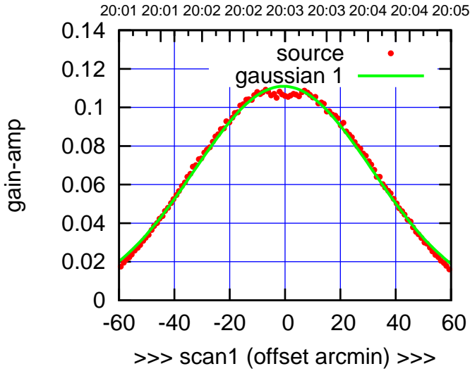
S03-130-AZ OFF= -0.9'
