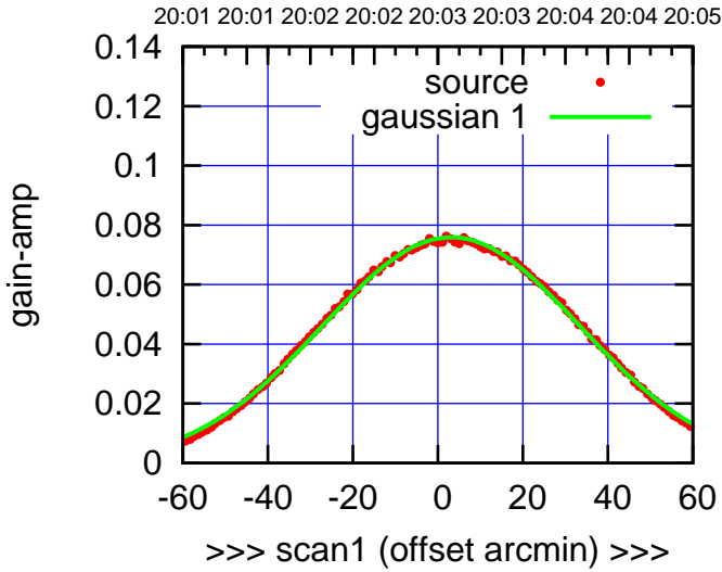
S04-130-AZ OFF= 2.8'
