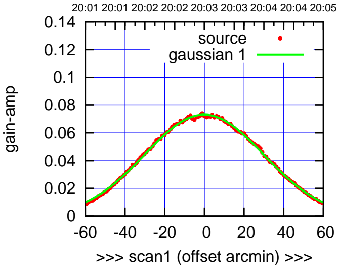
C03-130-AZ OFF= -0.7'
