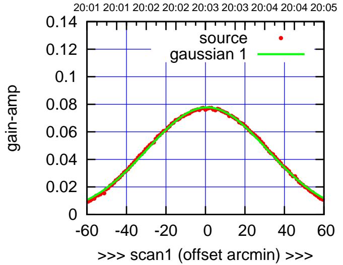
C09-175-AZ OFF= 0.4'
