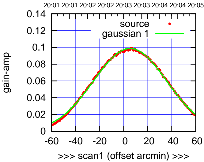
C04-130-AZ OFF= 5.4'
