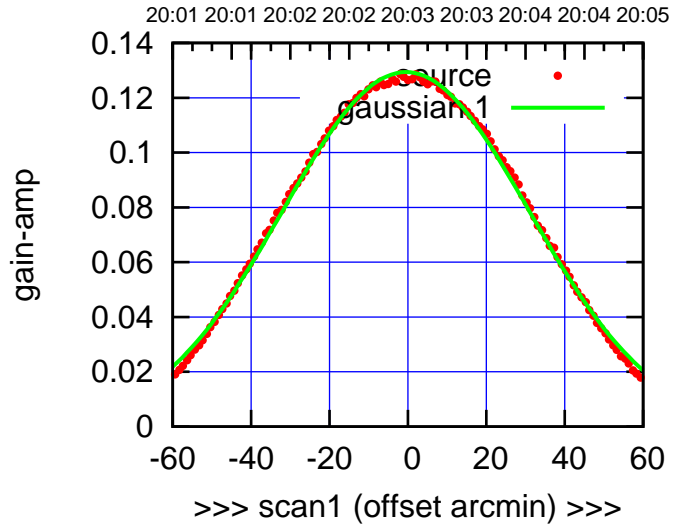
W01-175-AZ OFF= -1.0'
