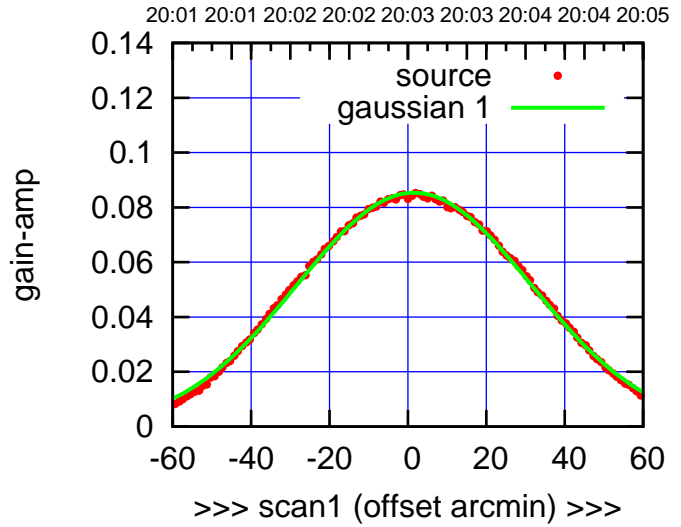
C08-175-AZ OFF= 1.6'
