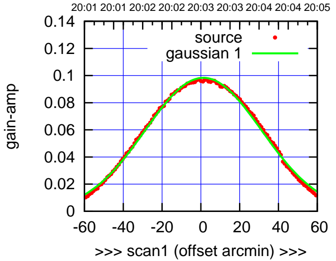
E05-175-AZ OFF= 1.1'
