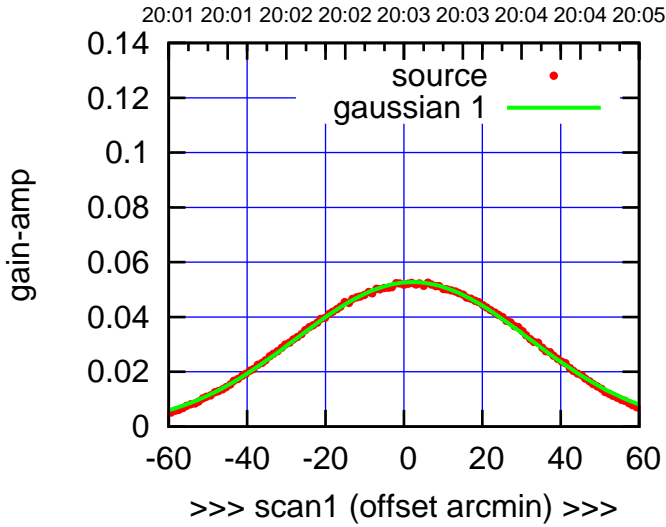
E03-130-AZ OFF= 1.8'
