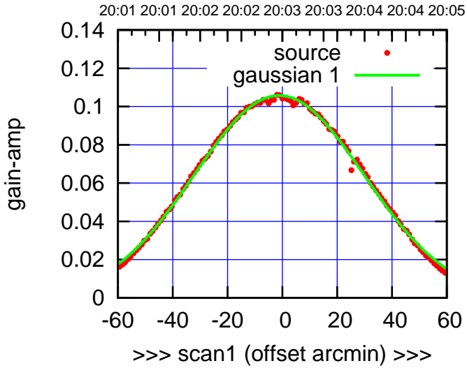
W04-130-AZ OFF= -1.8'
