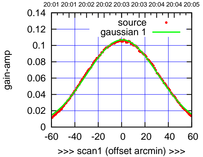
E04-175-AZ OFF= 0.4'
