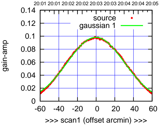
E04-130-AZ OFF= -0.4'
