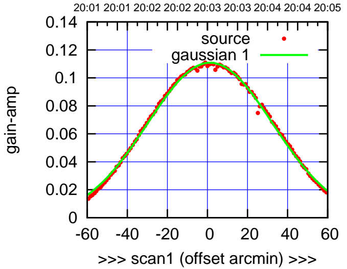
W04-175-AZ OFF= 0.6'
