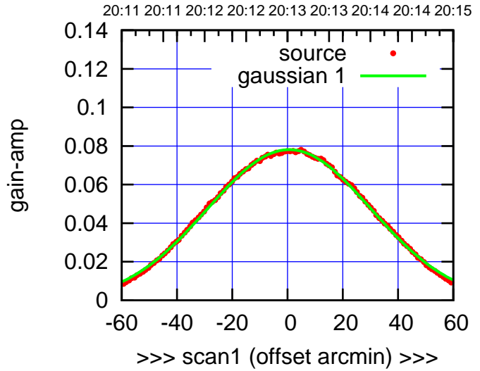
C09-175-AZ OFF= -0.1'
