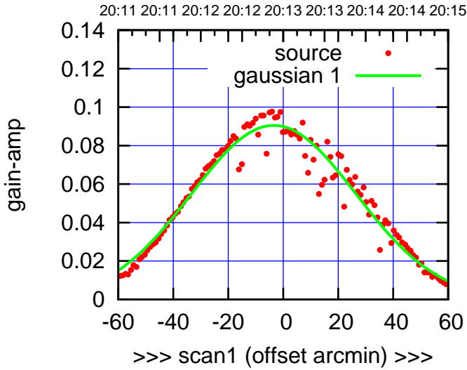
C14-130-AZ OFF= -1.7'
