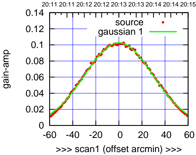
C11-130-AZ OFF= 0.1'
