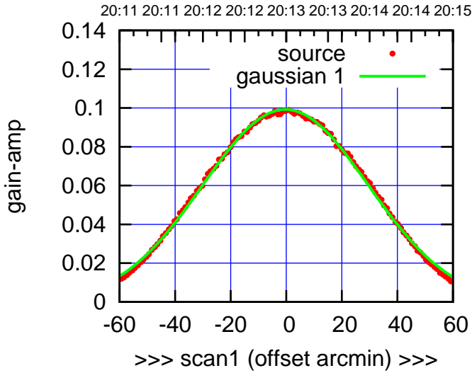
W03-130-AZ OFF= -0.2'
