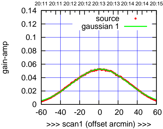
E03-130-AZ OFF= 1.6'
