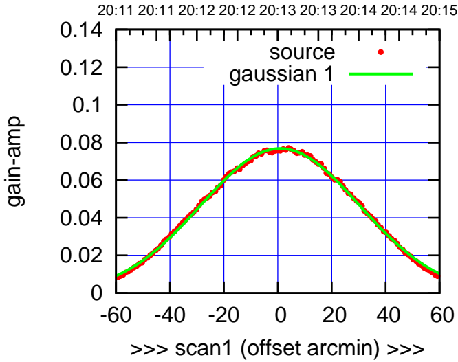
C09-130-AZ OFF= 0.0'
