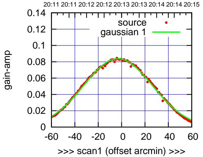
C01-175-AZ OFF= -2.5'
