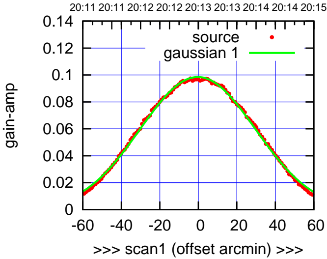
E04-130-AZ OFF= -0.8'
