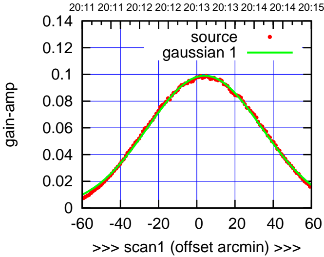
W06-130-AZ OFF= 4.0'
