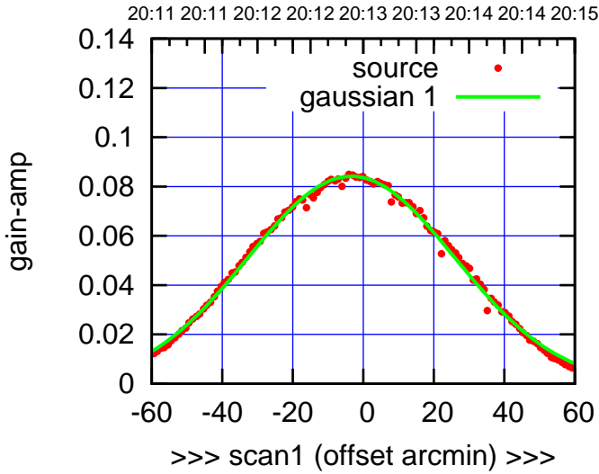
C01-130-AZ OFF= -2.6'
