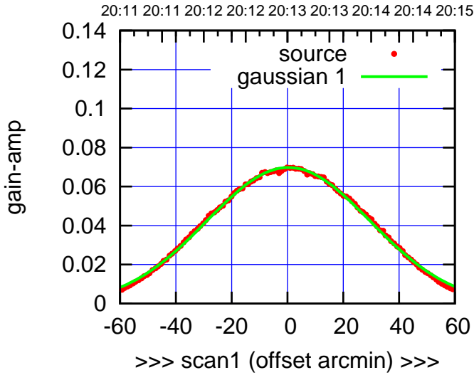
E05-130-AZ OFF= -0.1'
