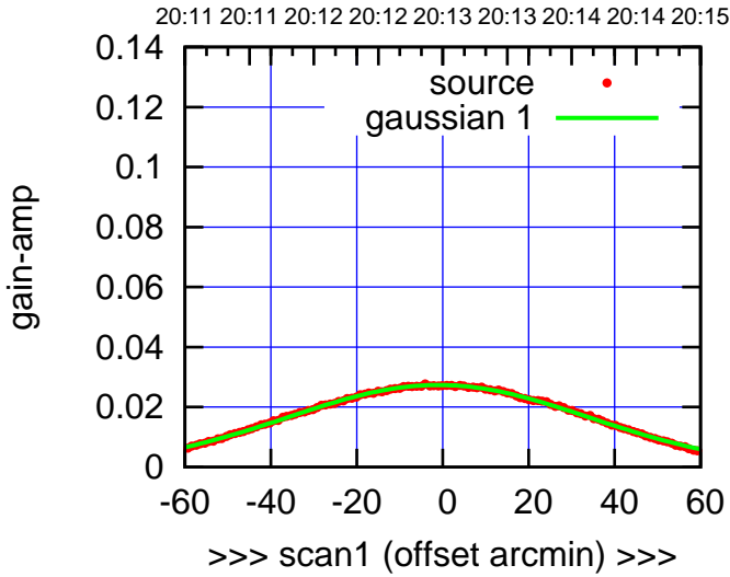
E06-130-AZ OFF= -2.6'
