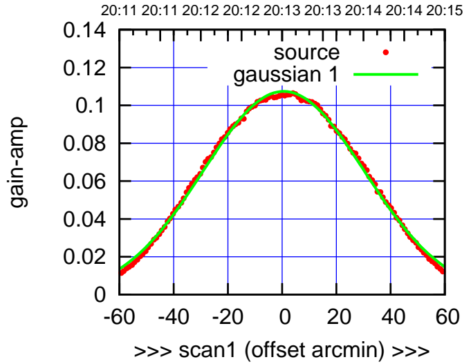
E04-175-AZ OFF= 0.1'
