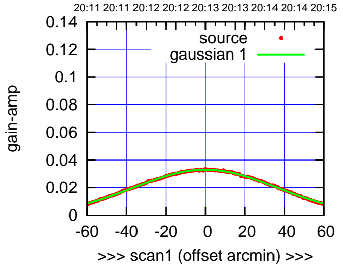
E06-175-AZ OFF= -1.6'
