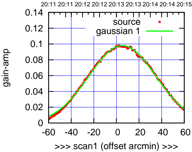
C04-130-AZ OFF= 4.7'
