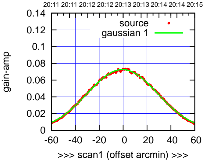
C03-130-AZ OFF= -0.9'
