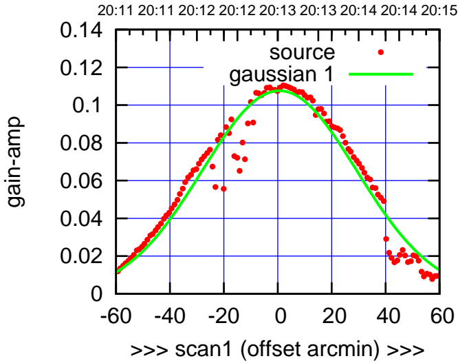
C06-130-AZ OFF= -3.2'
