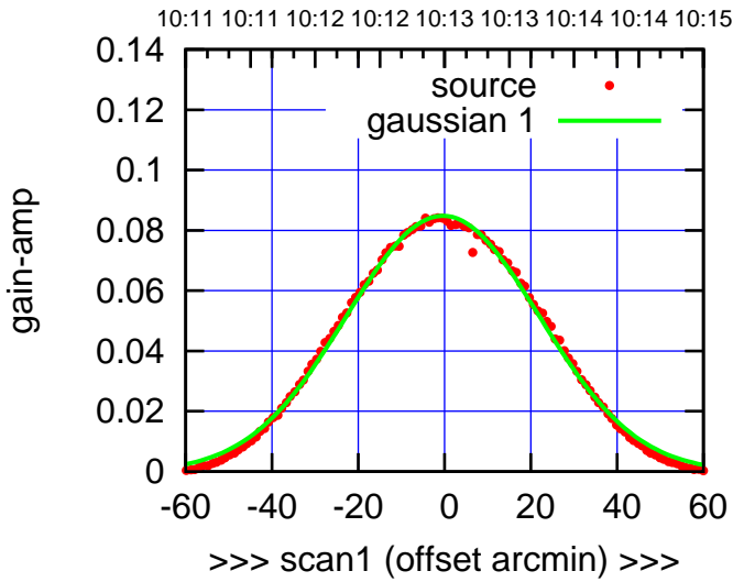
E04-130-AZ OFF= -0.9' ( 52.2')
