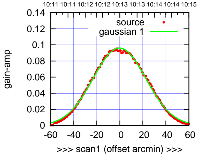
W01-175-AZ OFF= -0.7' ( 53.7')
