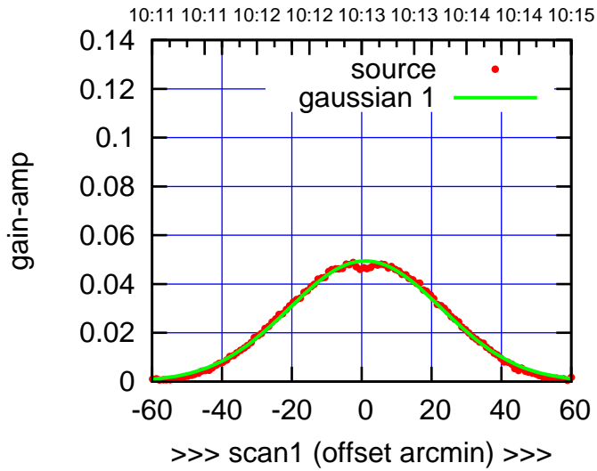
C13-130-AZ OFF= 1.0' ( 51.7')
