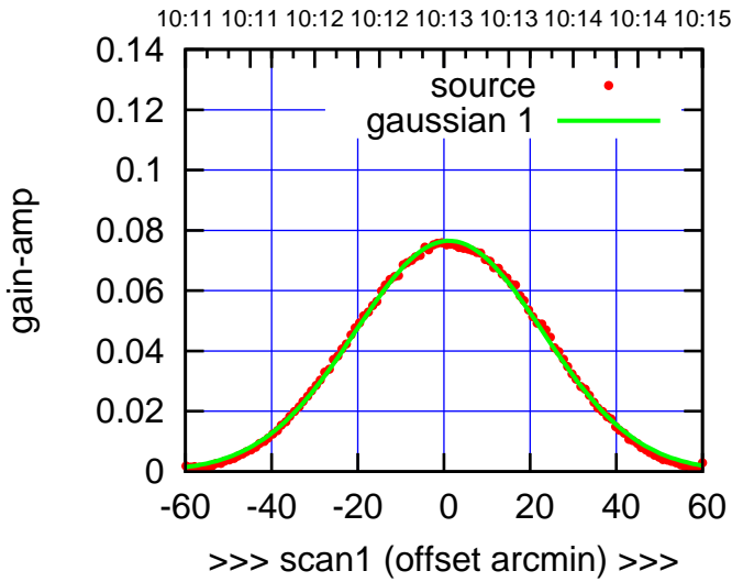
C05-130-AZ OFF= 0.4' ( 51.0')
