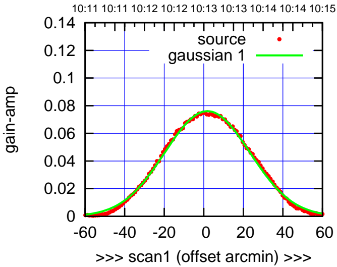
C14-130-AZ OFF= 1.4' ( 50.5')
