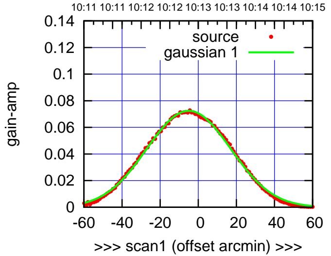
C01-175-AZ OFF= -5.3' ( 51.1')
