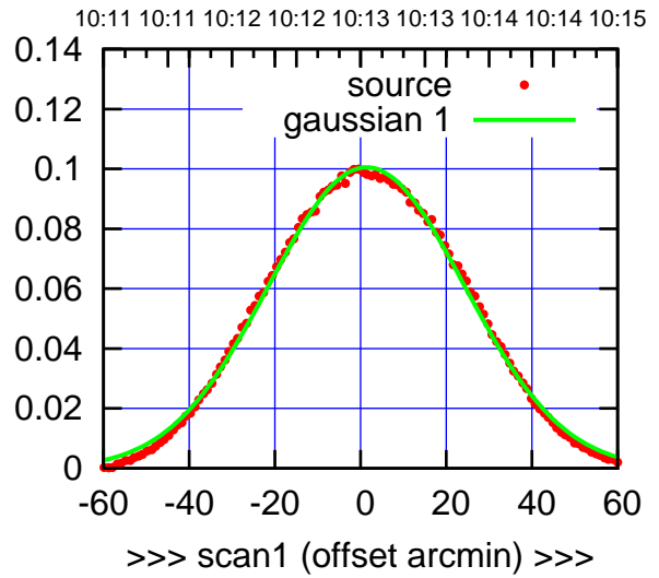
E06-175-AZ OFF= 0.8' ( 53.5')
