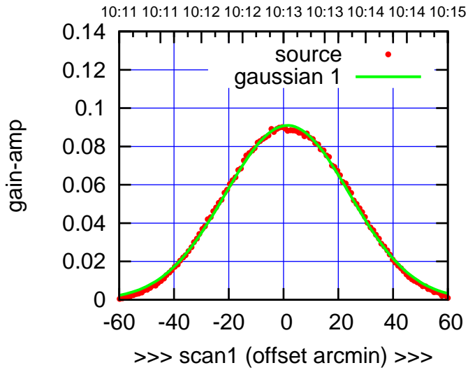
E02-130-AZ OFF= 0.4' ( 53.4')
