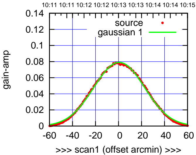
W03-130-AZ OFF= 0.3' ( 51.7')
