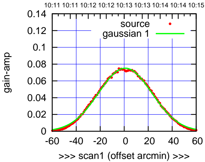
C04-130-AZ OFF= 0.7' ( 52.1')
