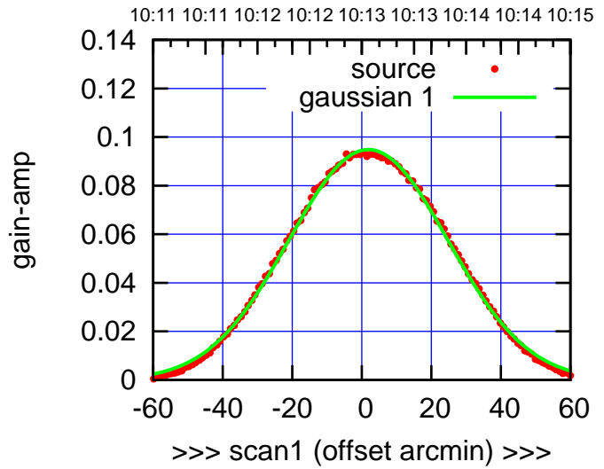
E02-175-AZ OFF= 1.0' ( 53.9')
