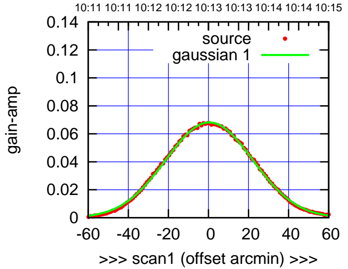
C03-175-AZ OFF= -0.3' ( 50.6')
