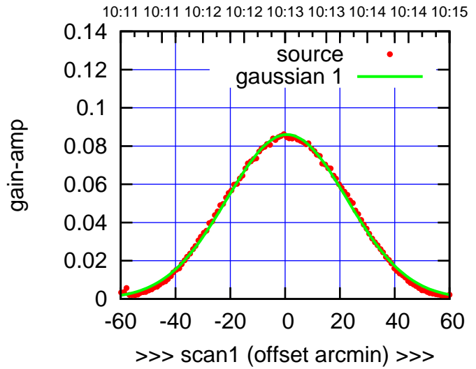
C08-175-AZ OFF= 0.4' ( 51.0')
