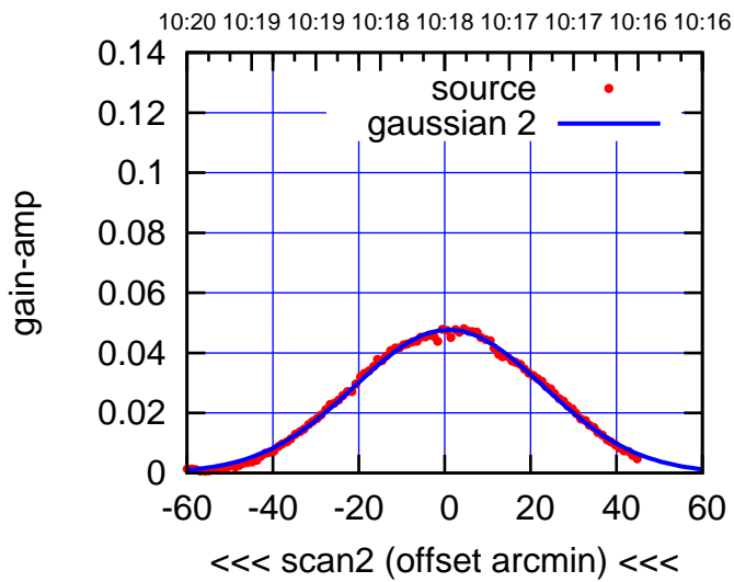
BACKLASH ERROR= 0.1'
