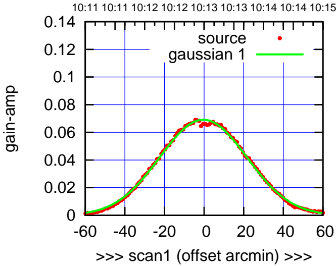
C03-130-AZ OFF= -1.2' ( 51.3')
