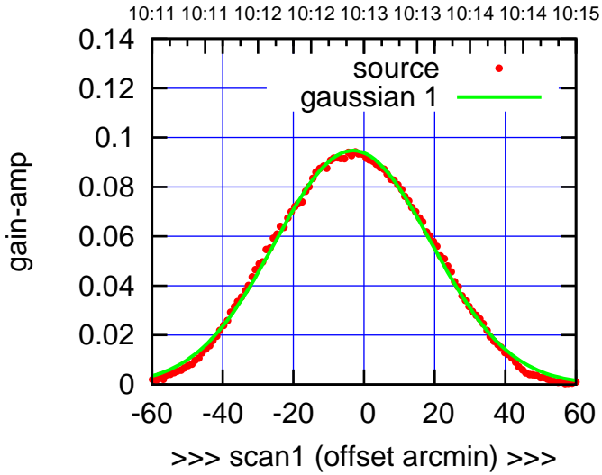
C06-130-AZ OFF= -3.9' ( 52.0')
