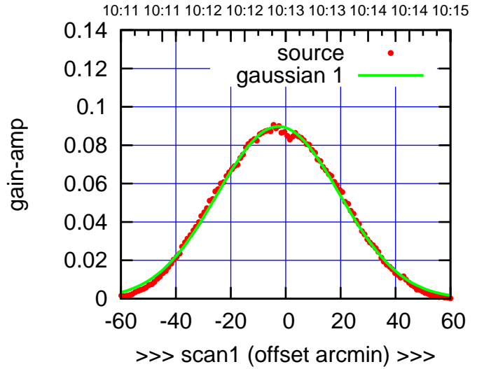
C06-175-AZ OFF= -3.2' ( 52.6')
