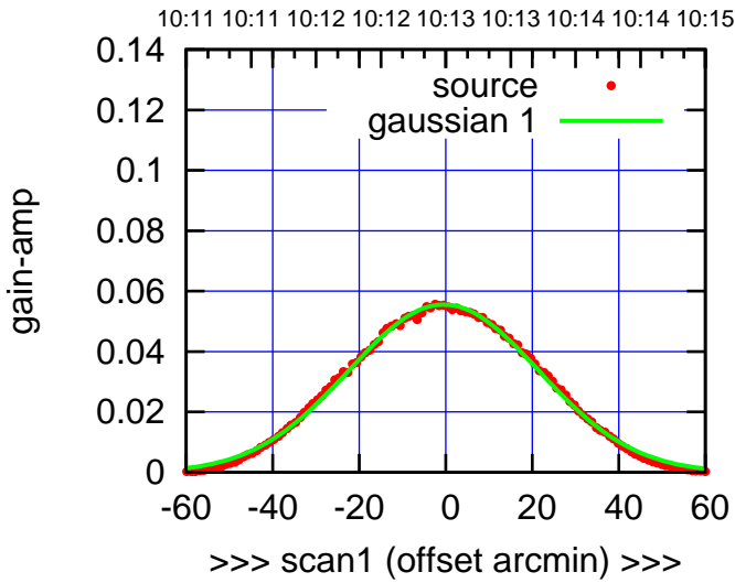
E05-130-AZ OFF= -1.0' ( 51.5')
