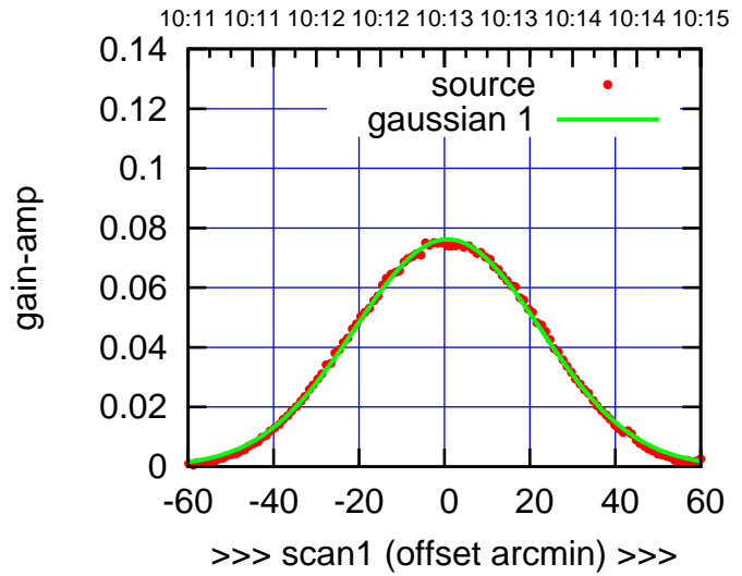
C05-175-AZ OFF= 0.1' ( 50.8')
