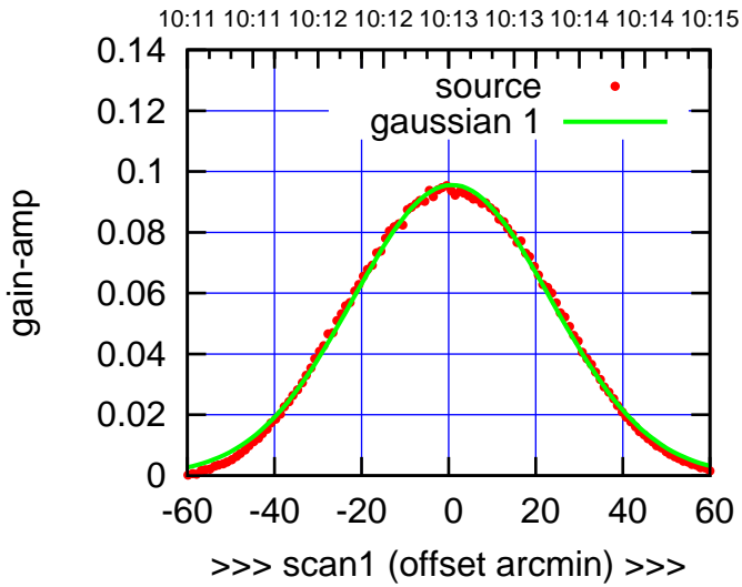
E06-130-AZ OFF= 0.1' ( 53.3')
