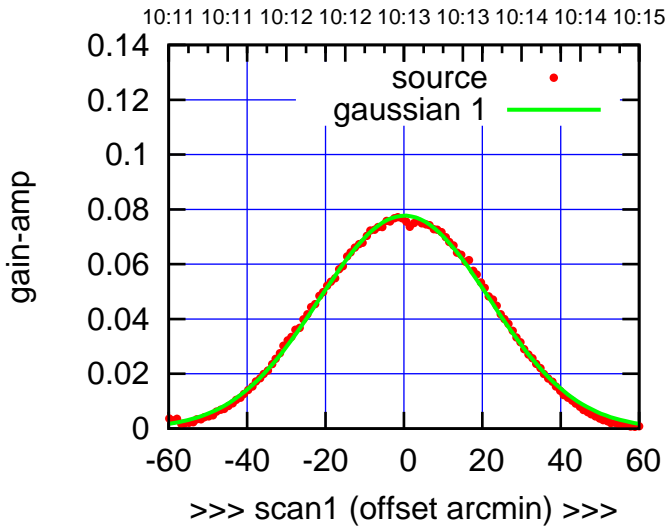
C08-130-AZ OFF= 0.0' ( 50.8')
