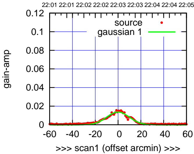
C05-130-EL OFF= -1.2' ( 24.3')
