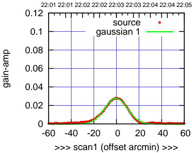
C06-130-EL OFF= -1.1' ( 23.4')
