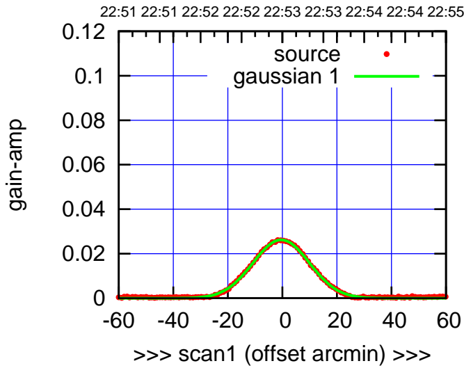
S02-130-AZ OFF= -1.0' ( 24.1')
