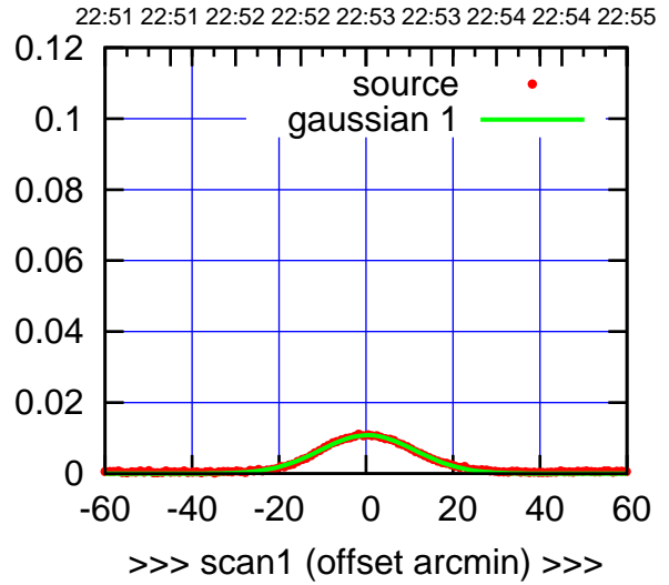
C10-175-AZ OFF= -0.1' ( 26.1')
