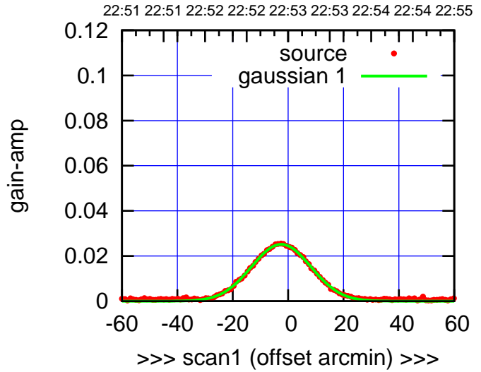
C02-175-AZ OFF= -2.8' ( 24.8')
