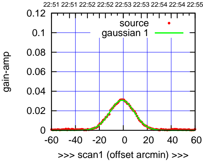
C04-130-AZ OFF= -1.8' ( 24.1')
