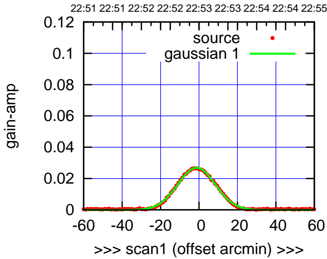
E02-130-AZ OFF= -2.2' ( 22.9')
