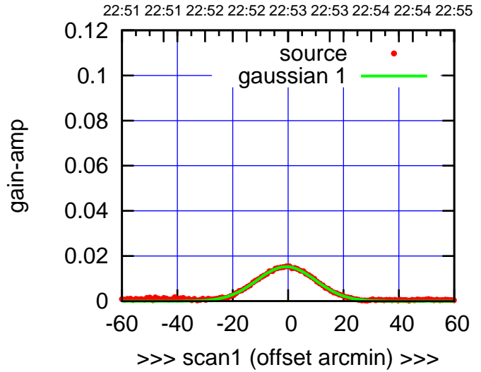
C01-175-AZ OFF= -1.5' ( 24.7')
