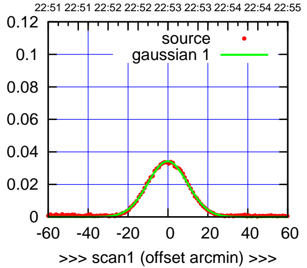
C08-175-AZ OFF= -0.5' ( 22.8')
