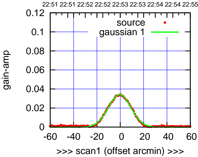
C08-130-AZ OFF= -0.8' ( 22.0')
