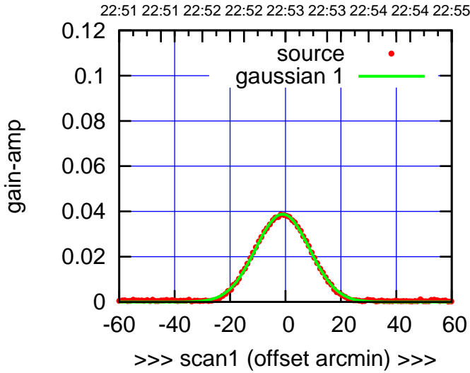
W03-130-AZ OFF= -1.7' ( 22.8')
