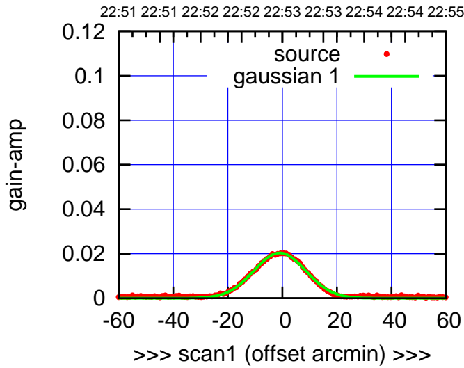
C03-130-AZ OFF= -2.0' ( 22.5')
