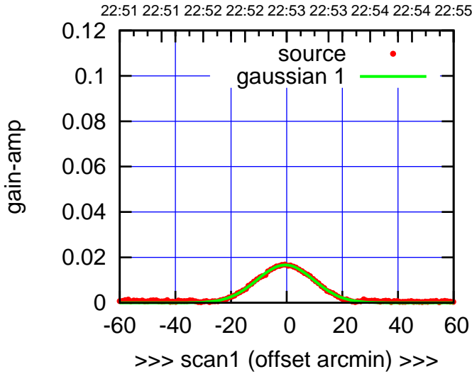
C01-130-AZ OFF= -1.3' ( 23.7')
