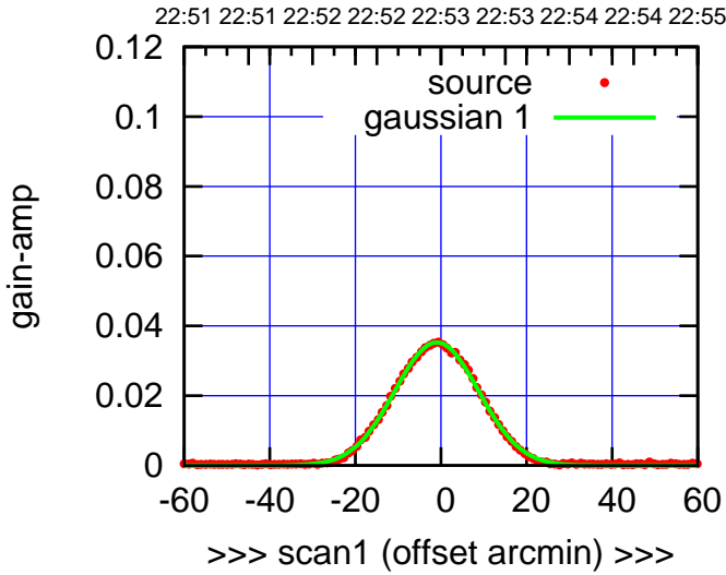
W05-130-AZ OFF= -1.1' ( 23.1')
