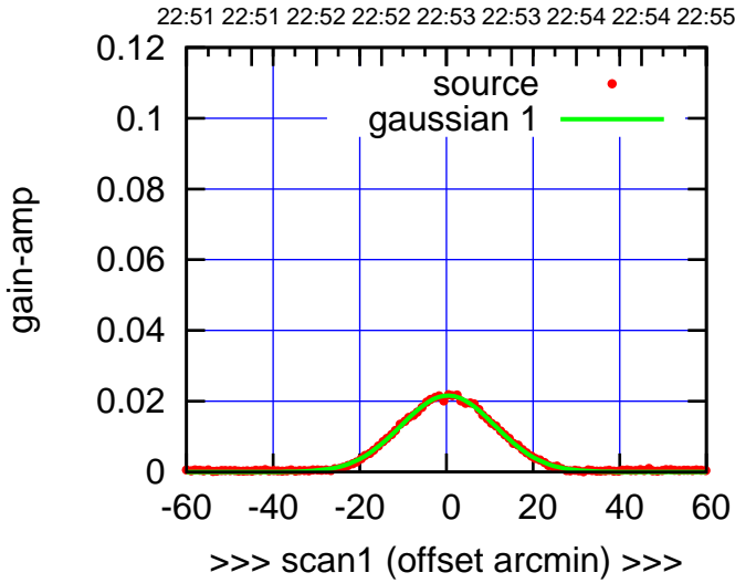
E03-130-AZ OFF= -0.2' ( 25.2')
