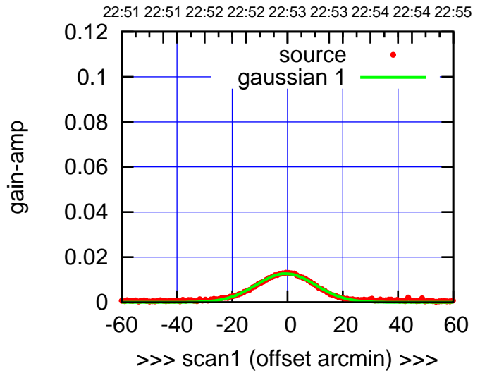
C03-175-AZ OFF= -1.7' ( 25.3')
