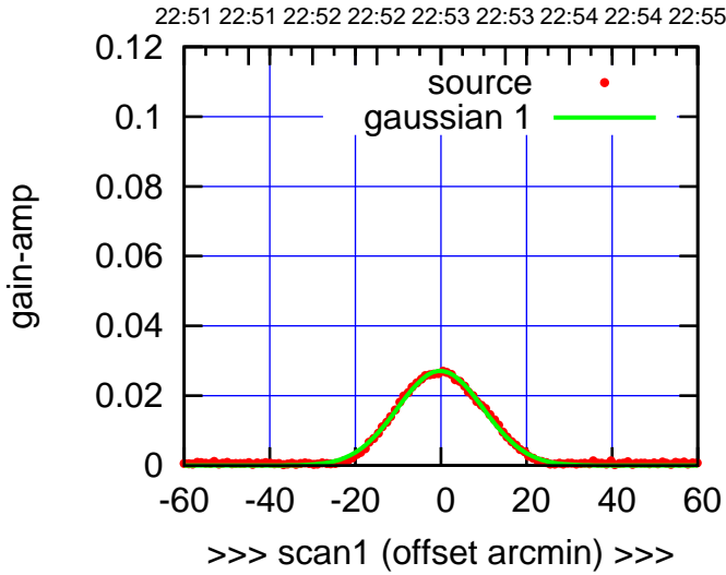
C06-130-AZ OFF= -1.4' ( 22.8')
