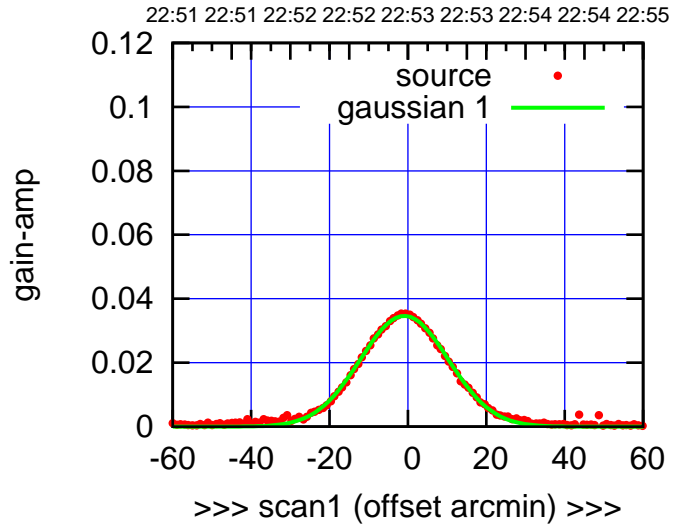
C04-175-AZ OFF= -1.2' ( 26.0')
