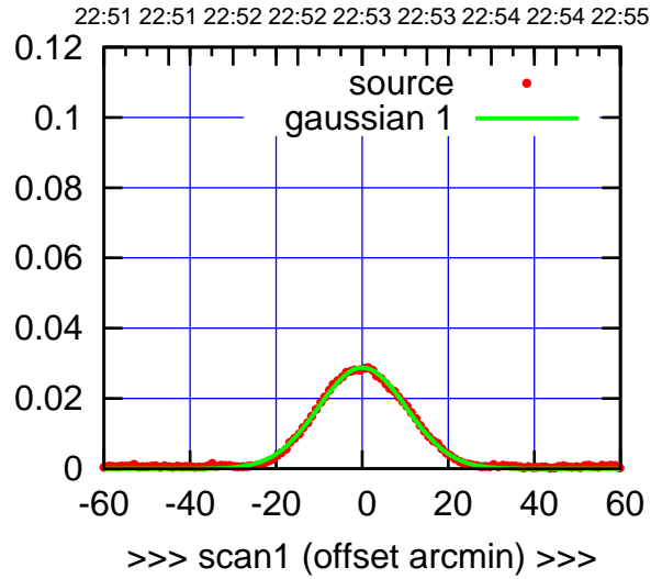
C06-175-AZ OFF= -1.1' ( 23.7')
