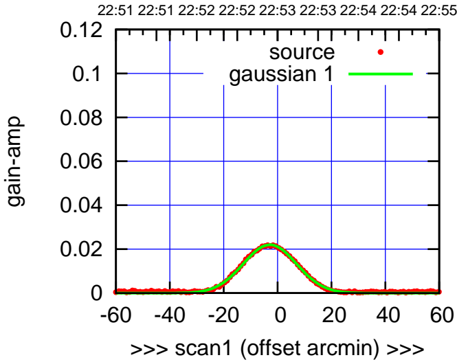
C02-130-AZ OFF= -3.1' ( 22.8')
