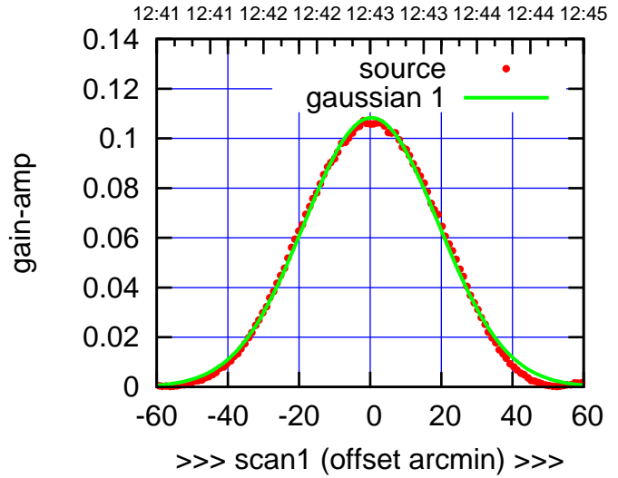
W04-175-EL OFF= 0.1'
