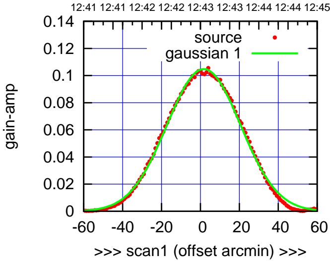
W04-130-EL OFF= 1.4'
