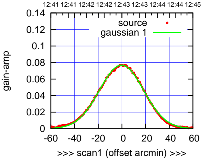
C03-130-EL OFF= -0.7'
